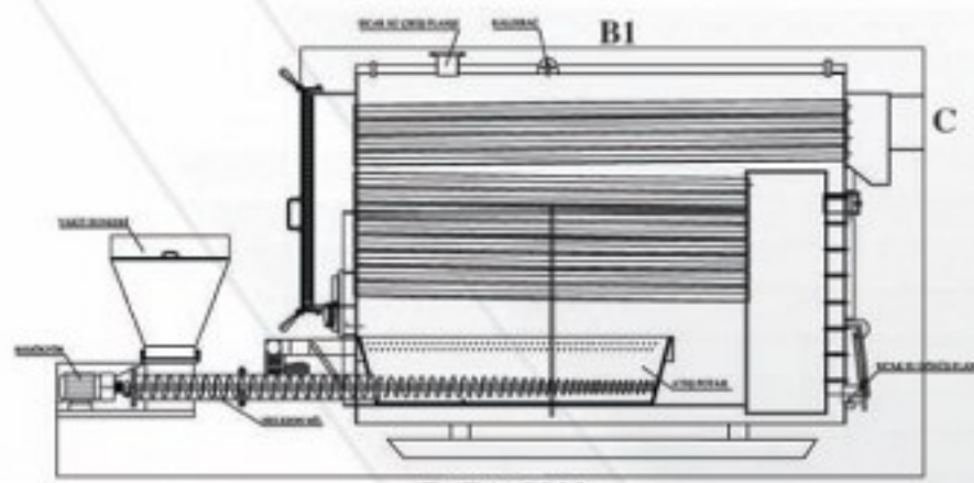
B=B1+2000mm YAN GÖRÜNÜŞ
