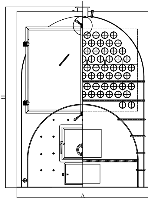
ÖN GÖRÜNÜŞ
