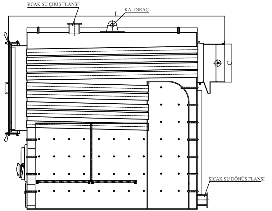
YAN GÖRÜNÜŞ
