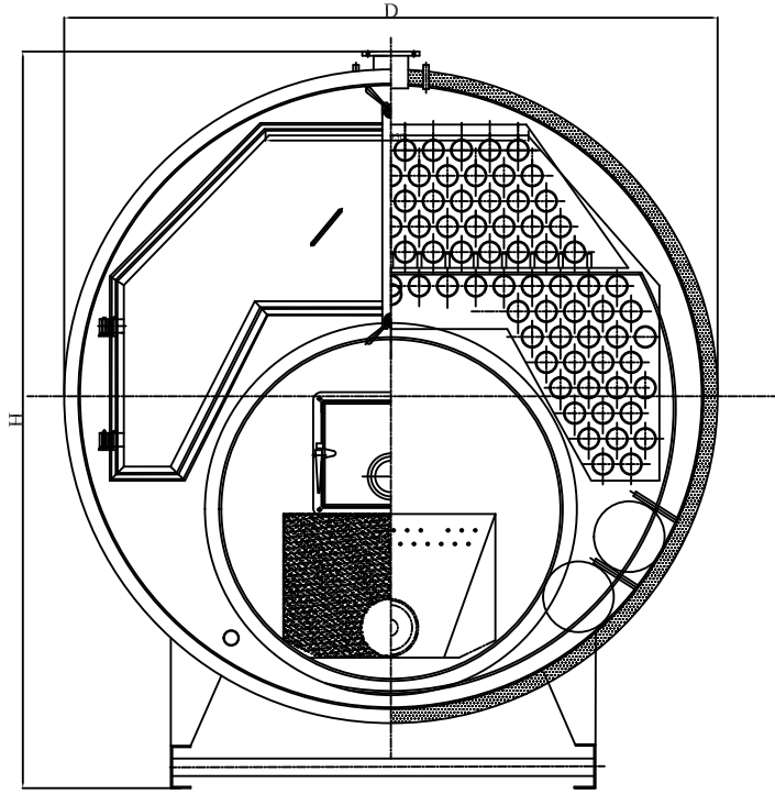
ÖN GÖRÜNÜŞ
