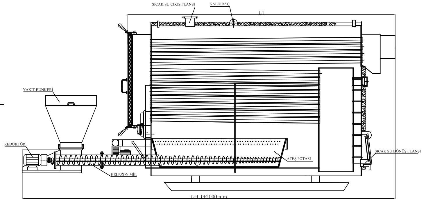
YAN GÖRÜNÜŞ
