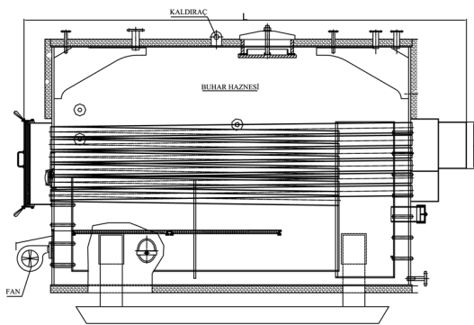
YAN GÖRÜNÜŞ
