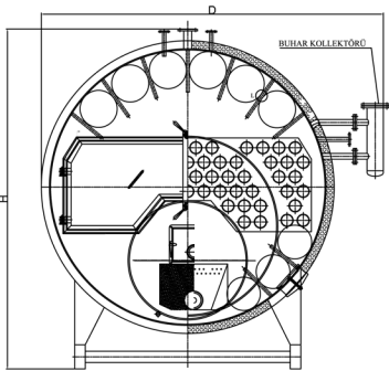
ÖN GÖRÜNÜŞ
