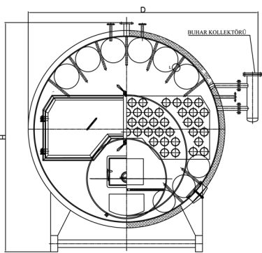
ÖN GÖRÜNÜŞ
